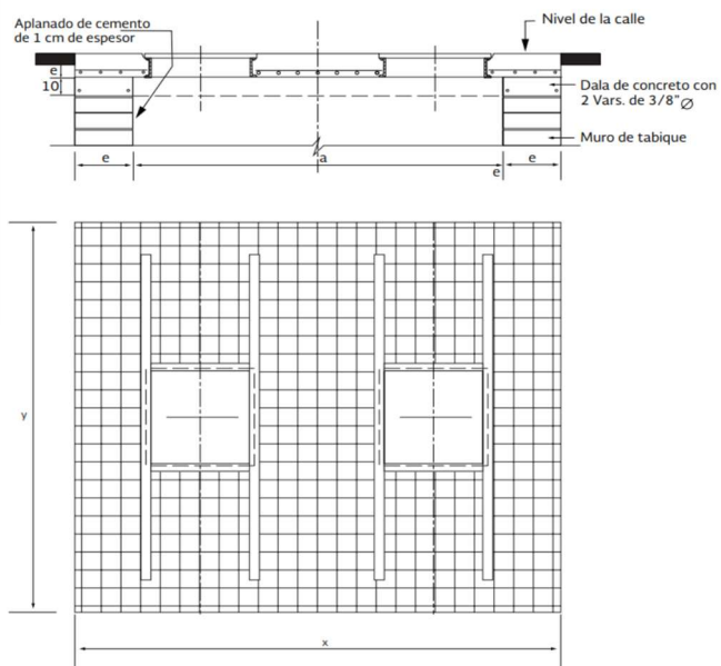
Caja Tipo 7
